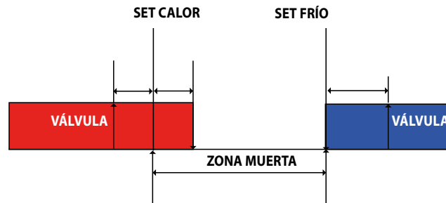
funcionamiento de integración fan coil y placa radiante
